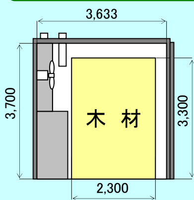
本体立面図
