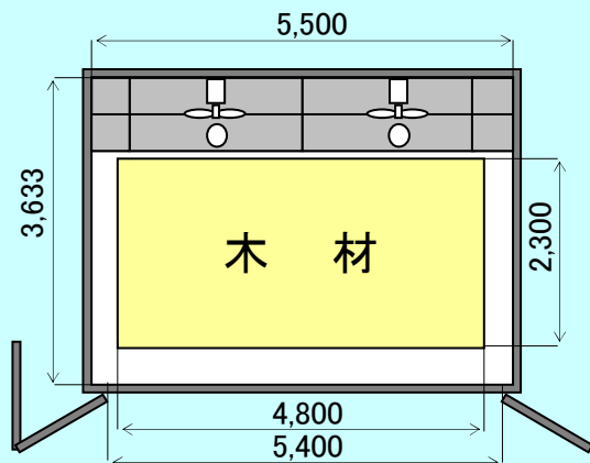
本体平面図
